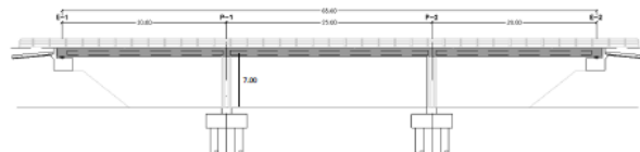
Figura 1 Alzado del paso superior
