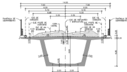
Figura 2. Sección transversal tipo del tablero
