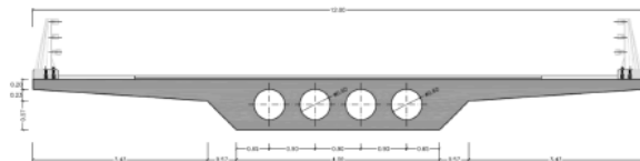
Figura 2 Sección del tablero
